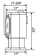
U38 & U39 SIDE
